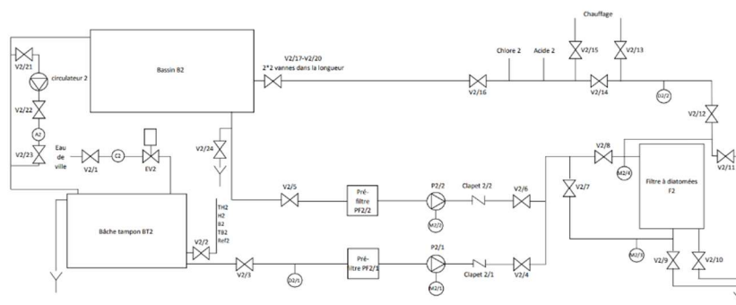
Schéma de procédé du grand bassin
