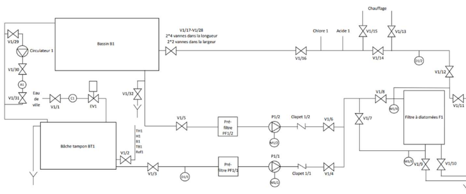
Schéma de procédé du grand bassin
